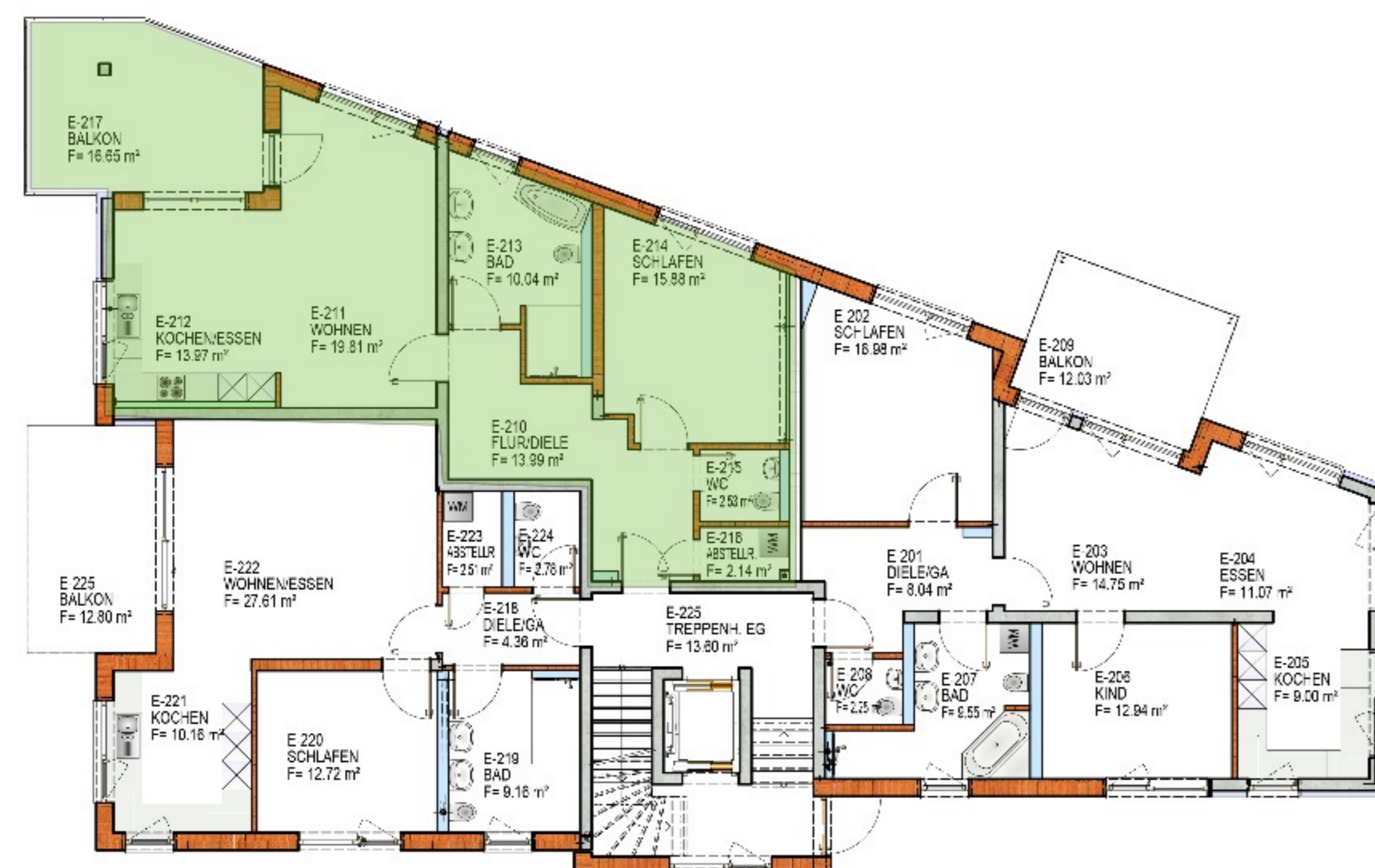
Erdgeschoss
